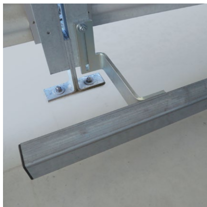
RAMMSCHUTZ Stahlrohr zum Schutz der Wandelemente vor Beschädigungen, beispielsweise durch Müllcontainer oder Fahrräder.
